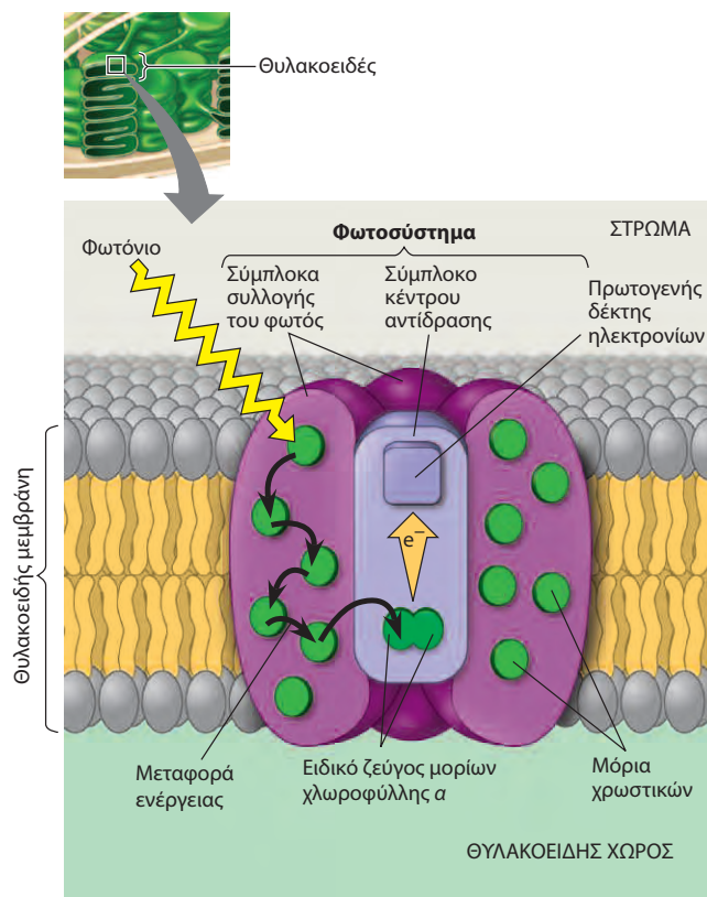
▲ Εικόνα 10.12 Συλλογή φωτονίων από ένα φωτοσύστημα. Όταν ένα φωτόνιο συναντήσει κάποιο μόριο χρωστικής του συμπλόκου συλλογής του φωτός, η ενέργειά του μεταφέρεται από μόριο σε μόριο μέχρι να φθάσει στο σύμπλοκο του κέντρου αντίδρασης. Εκεί, ένα διεγερμένο ηλεκτρόνιο μεταφέρεται από το ειδικό ζεύγος μορίων της χλωροφύλλης \alpha στον πρωτογενή ηλεκτρονιοδέκτη.
