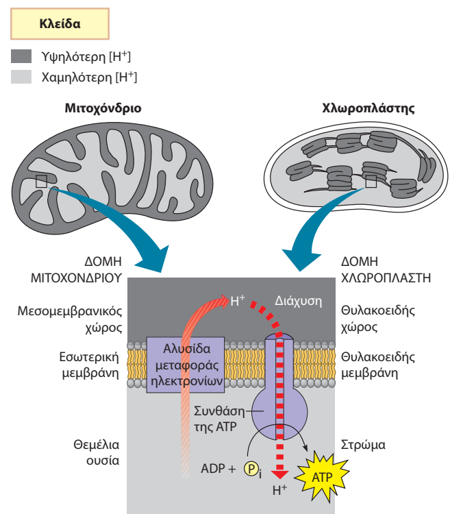
▲ Εικόνα 10.16 Σύγκριση της χημειώσωσης στα μιτοχόνδρια και στους χλωροπλάστες. Και τα δύο οργανίδια διαθέτουν αλυσίδες μεταφοράς ηλεκτρονίων που αντλούν πρωτόνια ( H^+ ) από την πλευρά της μεμβράνης με χαμηλή συγκέντρωση H^+ (ανοιχτό γκρίζο) προς την πλευρά με υψηλή συγκέντρωση H^+ (σκούρο γκρίζο). Κατόπιν, τα πρωτόνια διαχέονται σύμφωνα με τη διαβάθμιση της συγκέντρωσής τους και ξαναπερνούν από τη μεμβράνη. Επειδή όμως σε αυτή την πορεία κινούνται μέσω της δίοδου που τους παρέχει η συνθάση της ATP, θέτουν σε κίνηση τον μηχανισμό σύνθεσης ATP.
